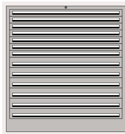
WSK 136 fiókos szekrény 7 db fiók 60/35 mm, 6 db fiók 90/65 mm.
