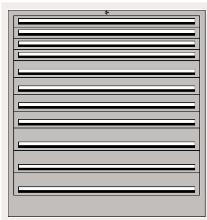
WSK 126 fiókos szekrény 4 db fiók 60/35 mm, 4 db fiók 90/65 mm, 3 db fiók 120/95 mm.
