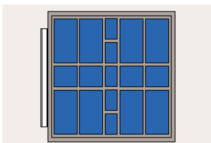
8 x EK 1, 4 x EK 2, 5 x EK 3 az SF 120-ban, SF 90-ben vagy az SF 180-ban
