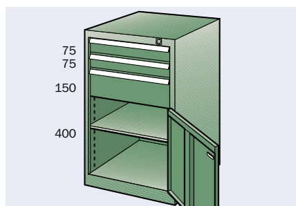
3 fiókkal*, 1 tálccával és ajtóval 1 áthelyezhető tálca, ajtó (400 mm magas).
