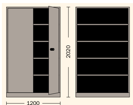
Szekrény, 1200 mm széles Lábazattal és 4 berakható polccal.
