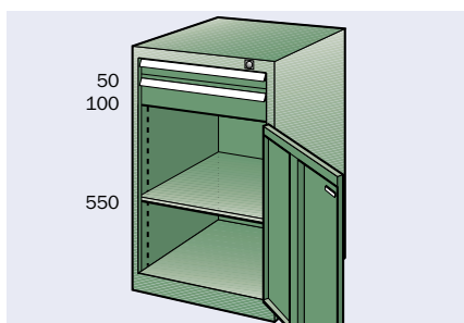
2 fiókkal*, 1 tálcával és ajtóval 1 áthelyezhető tálca, ajtó (550 mm magas).
