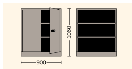
Alsó szekrény, 900 mm széles Lábazattal és 2 berakható polccal.
