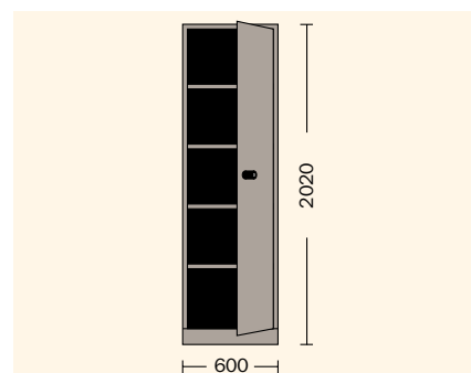
Szekrény, 600 mm széles Lábazattal és 4 berakható polccal.
