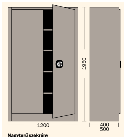
Nagyterű szekrény
