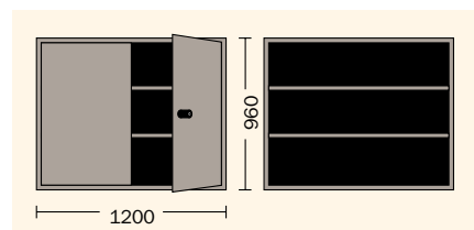
Rátétszekrény, 1200 mm széles Lábazat nélkül, 2 berakható polccal.
