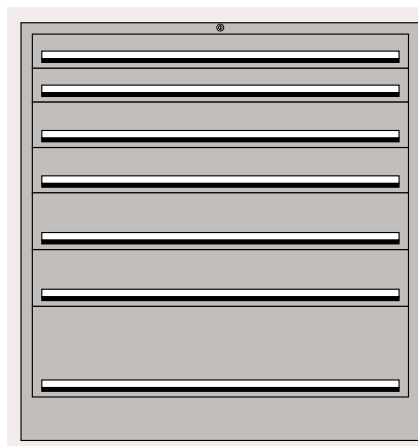
WSK 166 fiókos szekrény 2 db fiók 90/65 mm, 2 db fiók 120/95 mm, 2 db fiók 150/95 mm, 1 db fiók 240/95 mm.
