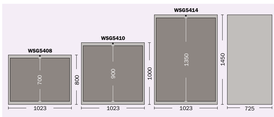
A WS 54 típus három különböző üres szekrényháza
