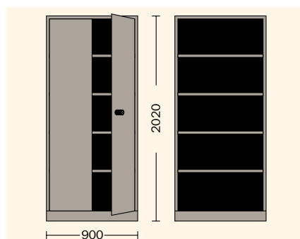
Szekrény, 900 mm széles Lábazattal és 4 berakható polccal.
