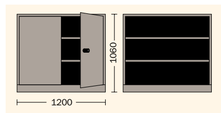
Alsó szekrény, 1200 mm széles Lábazattal és 2 berakható polccal.
