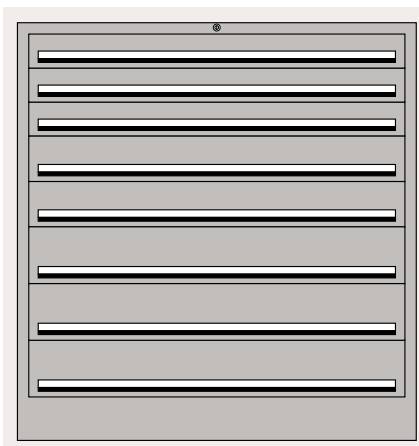
WSK 156 fiókos szekrény 3 db fiók 90/65 mm, 2 db fiók 120/95 mm, 3 db fiók 150/95 mm.
